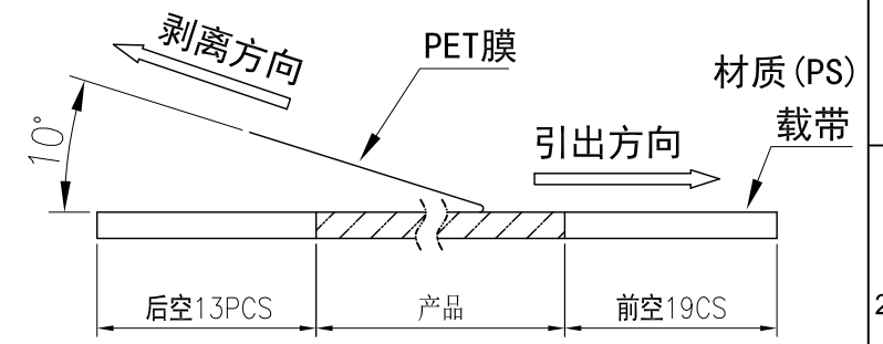
(PET膜剥离示意图)
